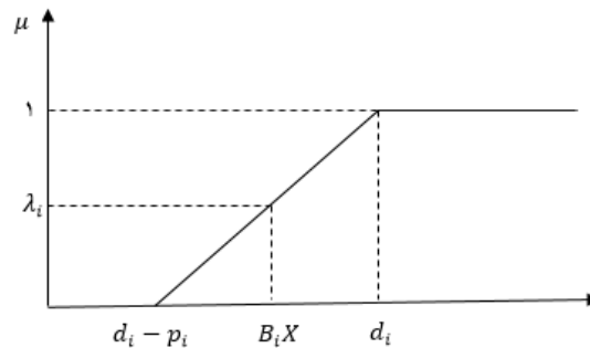
نمودار ۲: نمایش نموداری محدودیت فازی بزرگ‌تر مساوی
